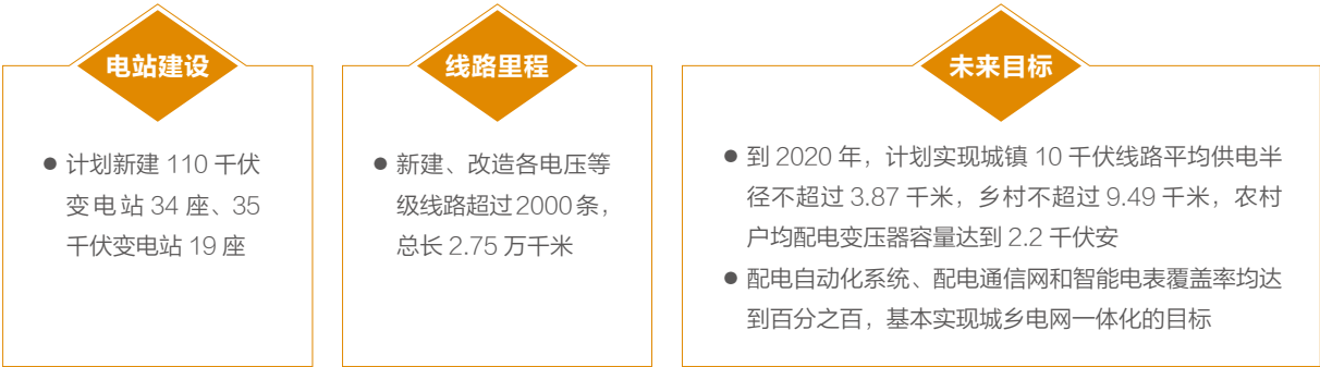
“十三五”农村电网建设规划
